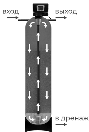
2. Прямая промывка
