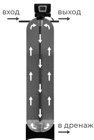
1. Обратная промывка
